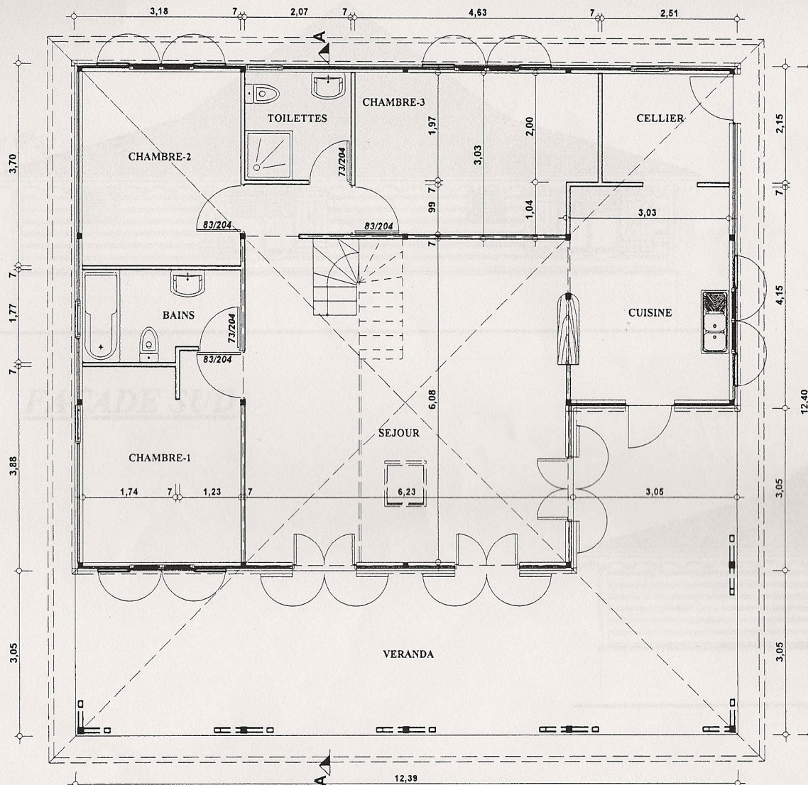
PLAN DU R.D.C.
