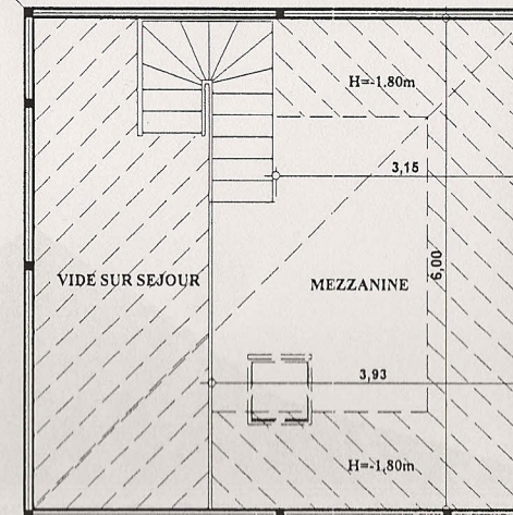
PLAN DE LA MEZZANINE
